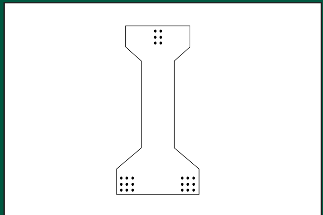
AASHTO I-BEAMS
