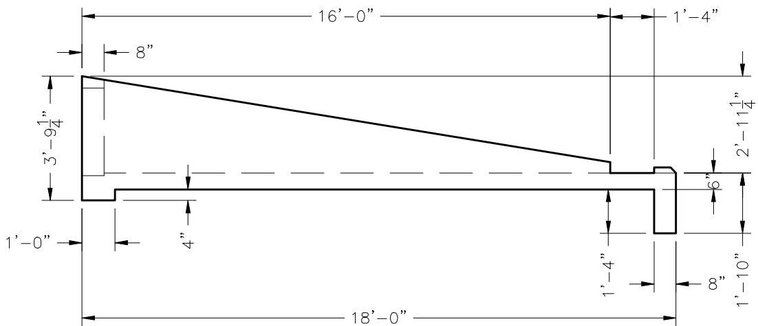
ELEVATION A-A
