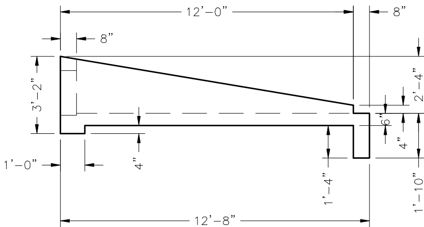
ELEVATION A-A
