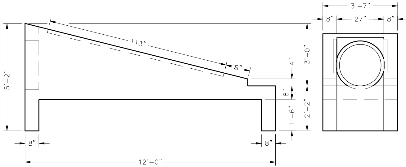
ELEVATION A-A
